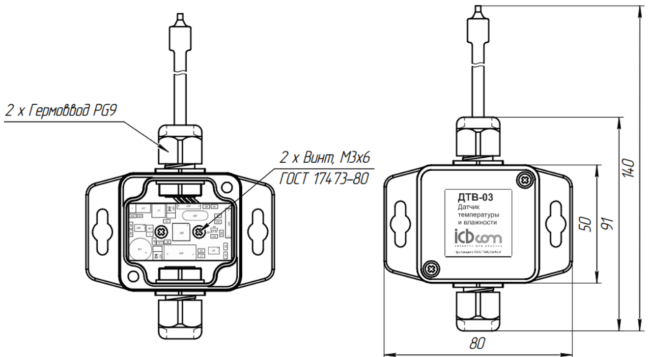
Рисунок 2 – Схема и габаритные размеры ДТВ-03
